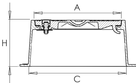
Coupe A-A
