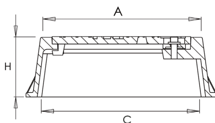
Coupe A-A
