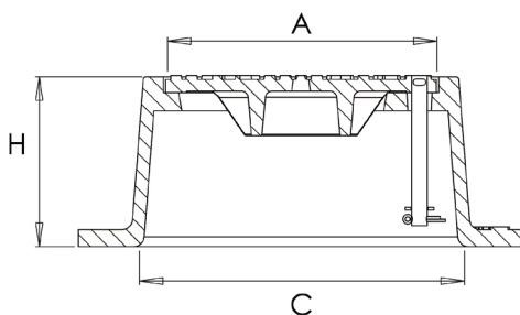
Coupe A-A
